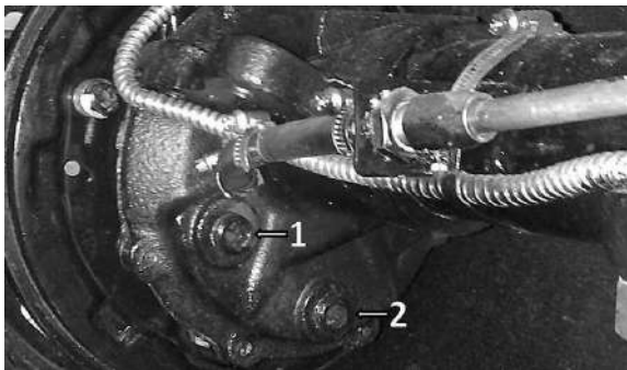
Рис. 9.6 Картер бортовой передачи: 1 - пробка заливного (контрольного) отверстия, 2 - пробка сливного отверстия
