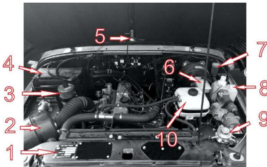
Рис. 4.1 Подкапотное пространство:
